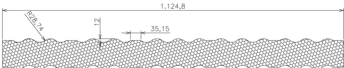
Figura 3 Sección transversal del panel MK2 entero.
