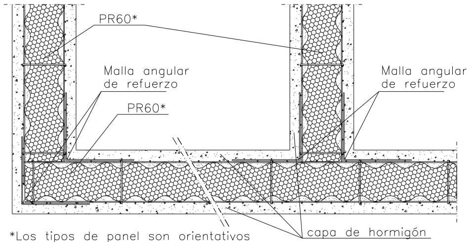
Figura 8 Detalle de encuentro entre muros (planta).
